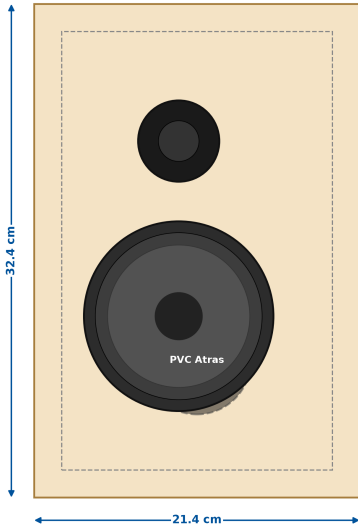
Caja Derecha (R)
