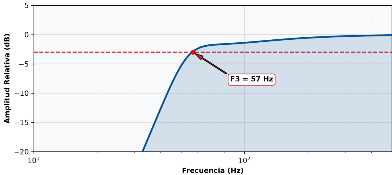
Respuesta de Frecuencia Simulada - Bass Reflex (PVC)
