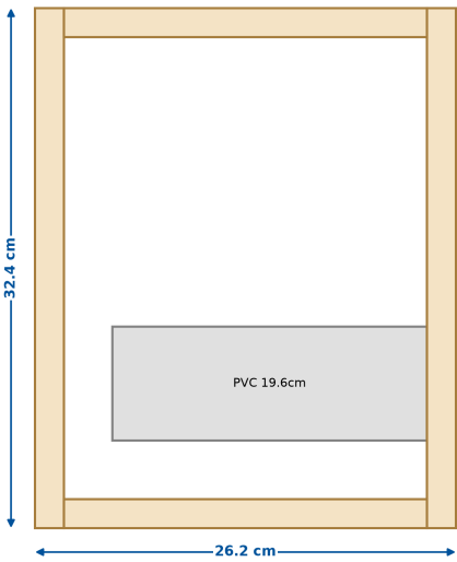
Corte Lateral (Ensamblaje)
